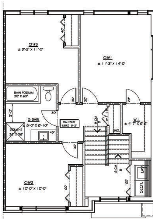
ÉTAGE 3 SUP. TOTALE: ± 754 pi.ca.
