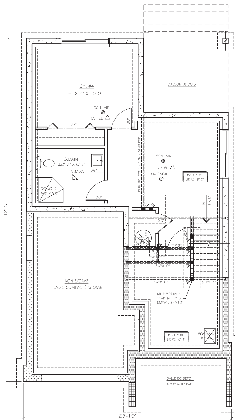
Sous-sol
