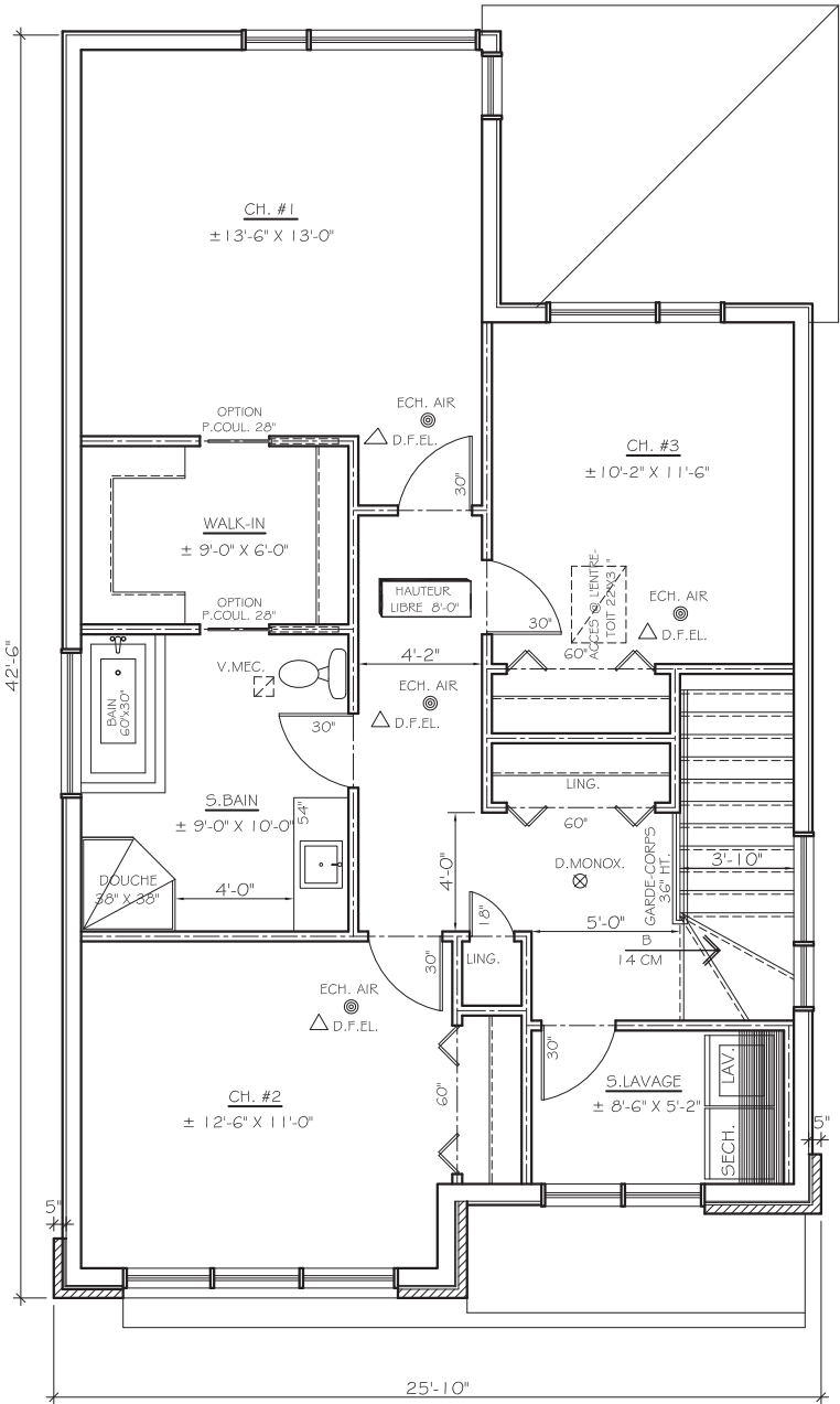
Étage
