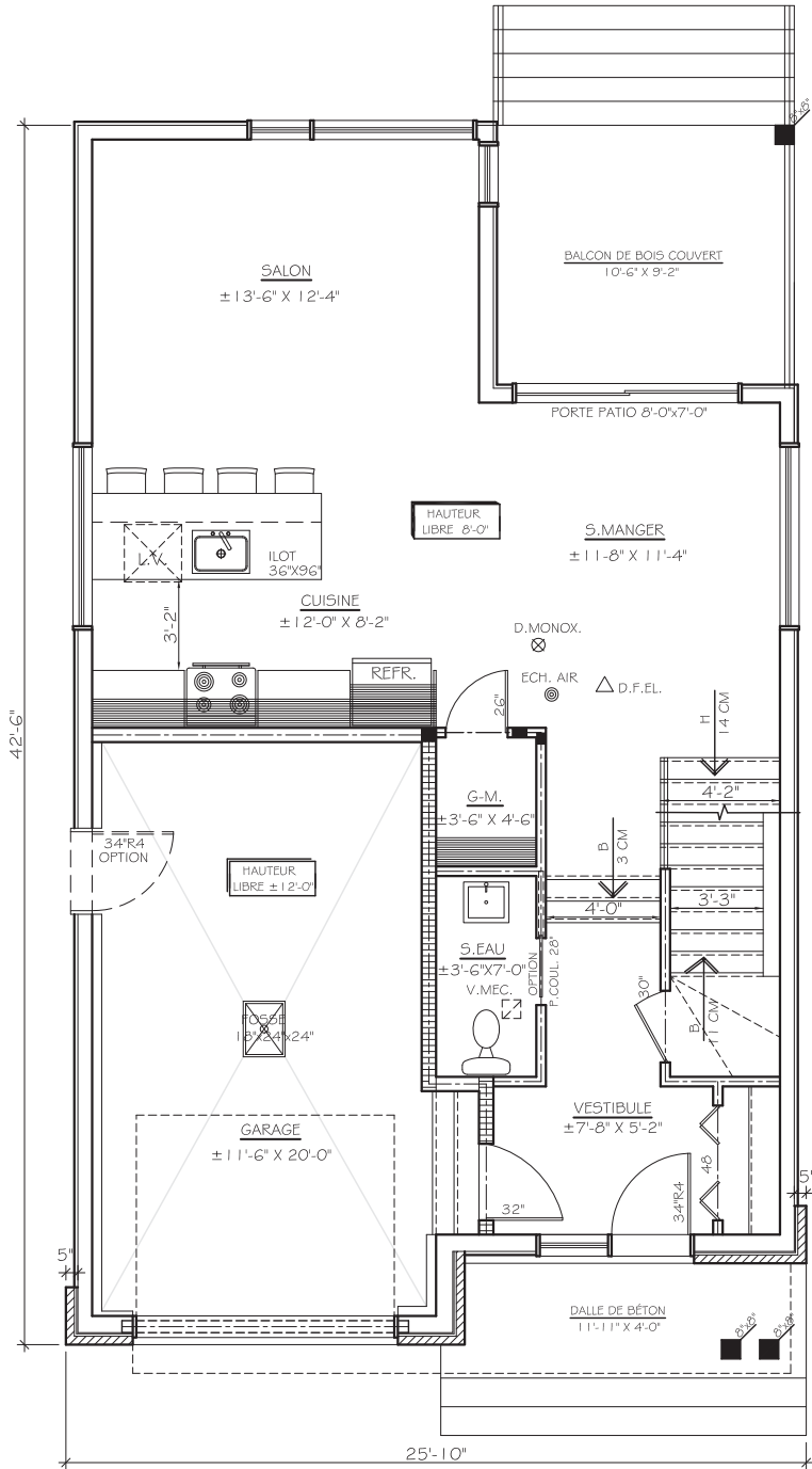
Rez-de-chaussée
