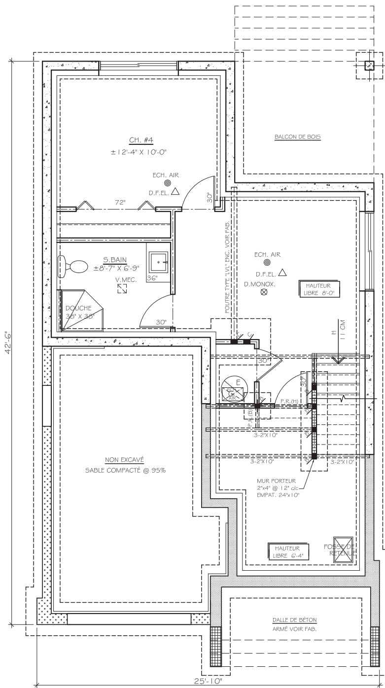
Sous-sol
