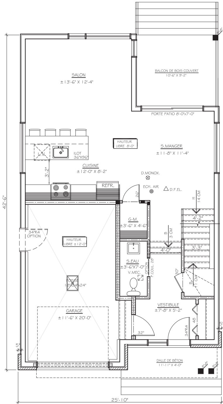
Rez-de-chaussée
